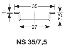
NS 35/7,5
