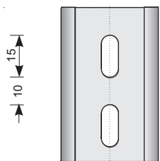
NS 35/15
