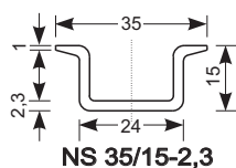
NS 35/15-2,3
