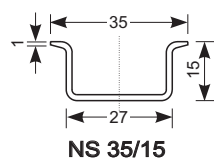
NS 35/15
