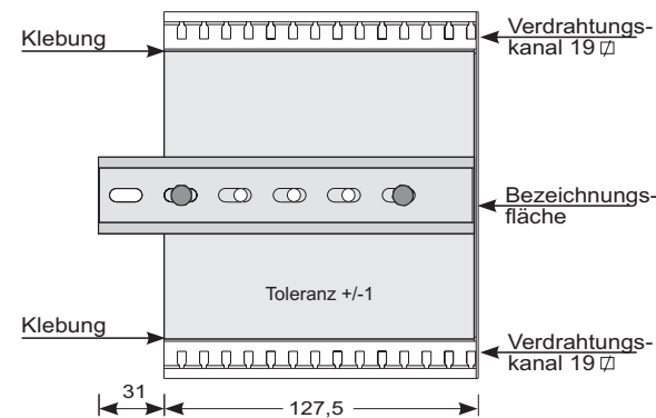
Montageteil M 125 (ES/DS)
