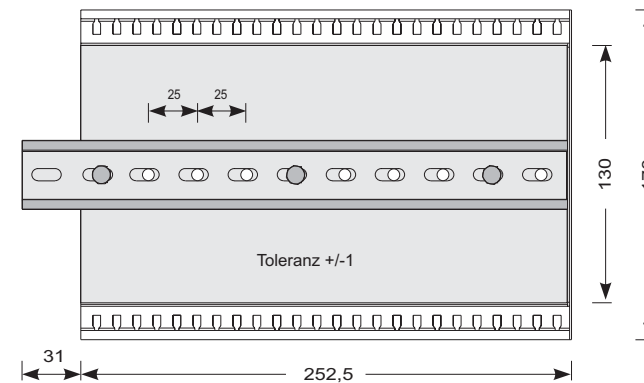
Montageteil M 250 (ES/DS) ABB. 2
