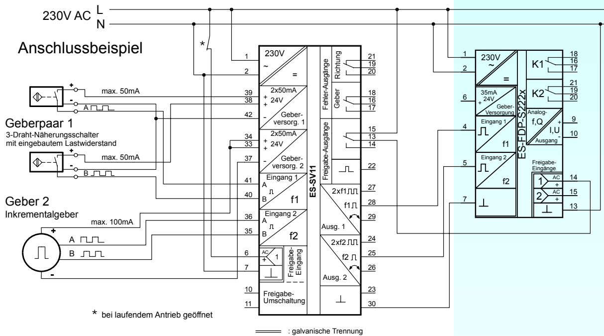
Bild 1: Anschlussbeispiel für eine Überwachung mit ES-SV11.2 und ES-FDP-S222x
